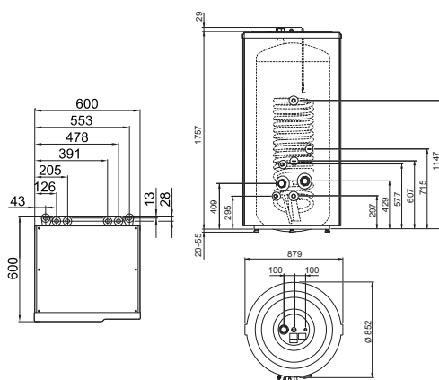
NIBE VPB 500
