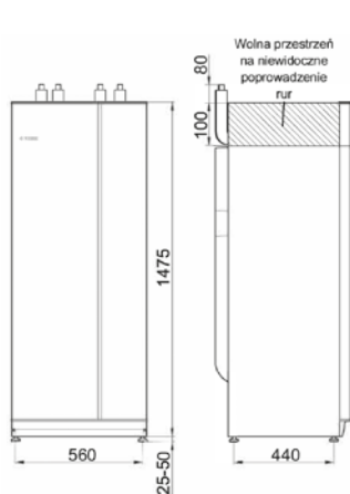
NIBE VPB 200
