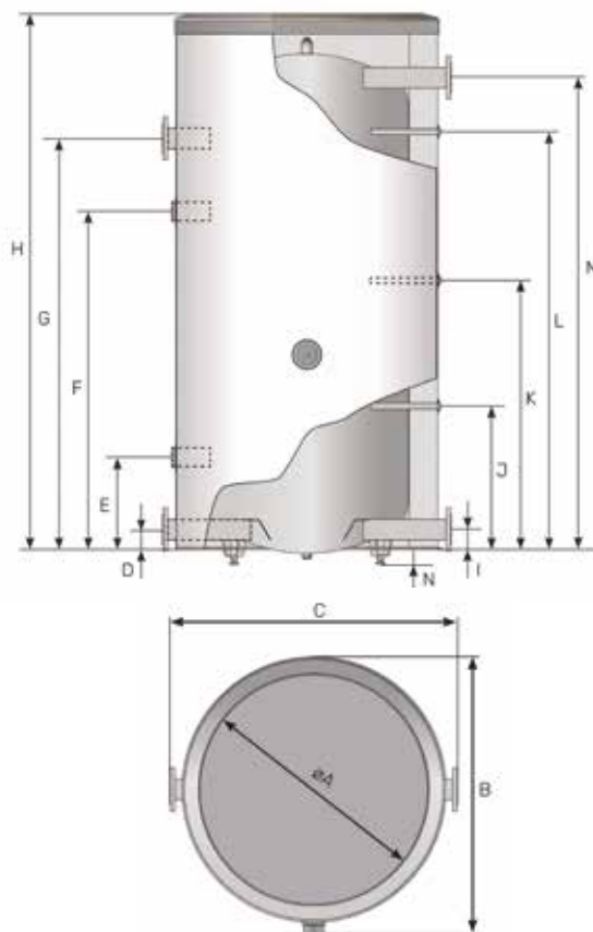
Przyłącze kołnierzowe DN80 (BU-1000.8 F) Typ 01 B PN6 EN 1092-1.
