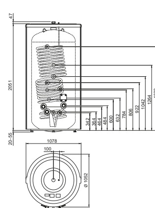
NIBE VPB 1000
