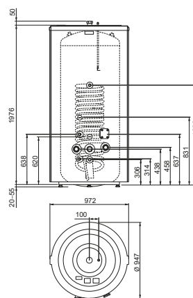
NIBE VPB 750
