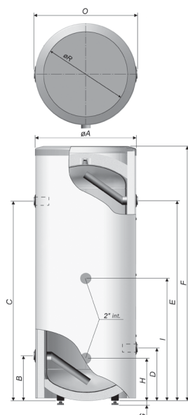
NIBE UKV 20-750/1000
