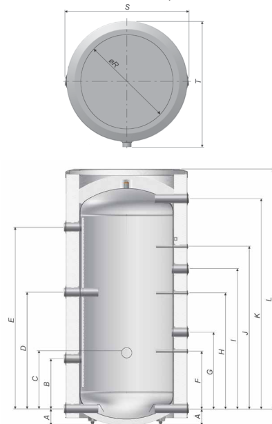
NIBE UKV 20-750/1000
