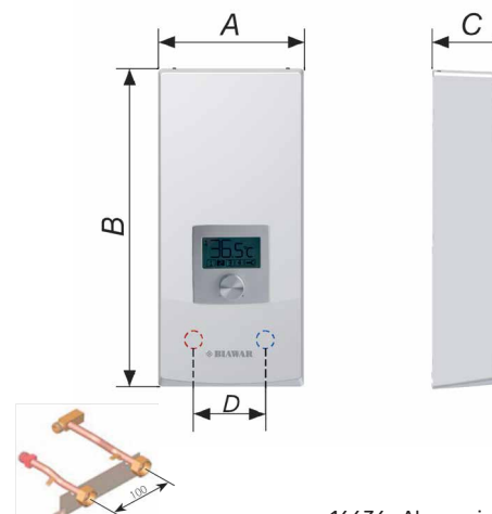
16636- Akcesorium, zespół przyłączeniowy od dołu, OP-xx.06, OP-xx.07
