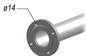
Przyłącze kołnierzone DN65 (BU-750.8 F) Typ 01 B PN6 EN 1092-1.
