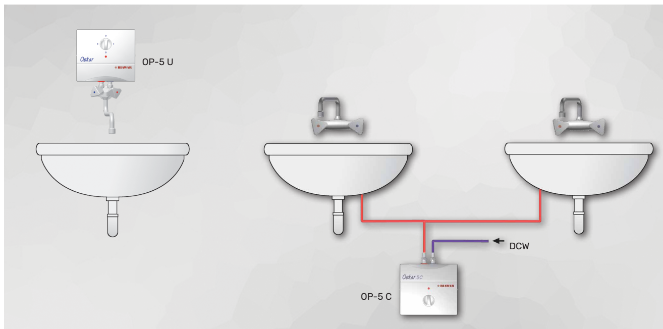
Przykładowe zastosowanie podgrzewaczy przepływowych OSKAR.
