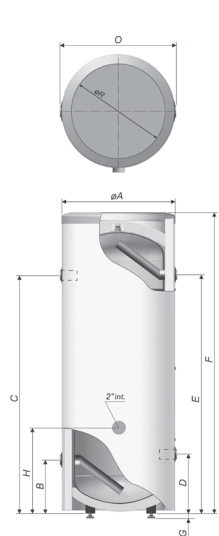
NIBE UKV 20-220
