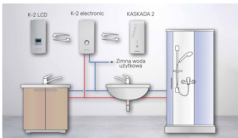
Przykładowe schematy hydrauliczne z podgrzewaczami KASKADA 2, K-2 electronic i K-2 LCD.
