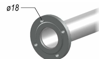
Przyłącze kołnierzone DN80 (BU-1000.8 F) Typ 01 B PN6 EN 1092-1.
