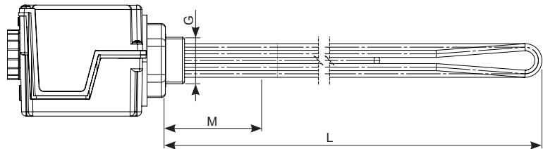
Рис. 10. Нагревательный модуль ME 0040 / ME 1045 / ME 1060 / ME 1090 / ME 2090 / ME 2120 / ME 2180.
