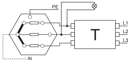
Rys. 5 Schemat elektryczny ME 0040 - ME 2090.
