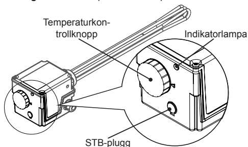
Ritning. 8 Framsidan på elpatroner ME 0040 / ME 1045 / ME 1060 / ME 1090 / ME 2090 / ME 2120 / ME 2180.
