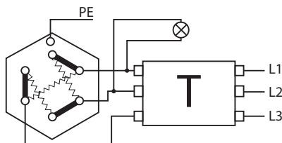
Рис. 6 Электрическая схема ME 2120 - ME 2180.
