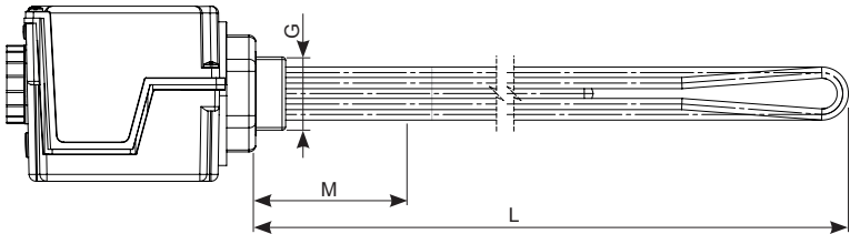
Rys. 10. Moduły grzejne ME 0040 / ME 1045 / ME 1060 / ME 1090 / ME 2090 / ME 2120 / ME 2180.
