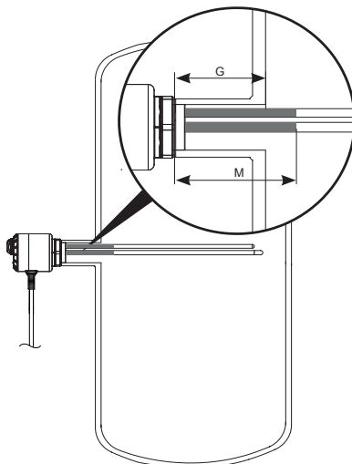
Rys. 3 Poprawna głębokość króćca przyłączeniowego.
