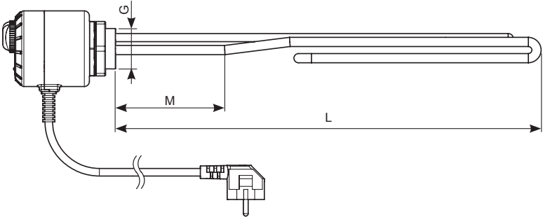
Rys. 9. Moduł grzejny ME 1030.
