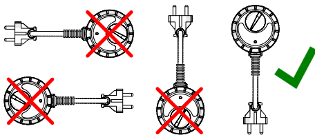
Rys. 4 Poprawny montaż modułu grzejnego.
