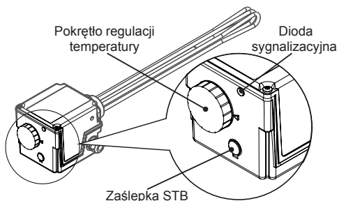
Rys. 8 Przód obudowy modułów grzejnych ME 0040 / ME 1045 / ME 1060 / ME 1090 / ME 2090 / ME 2120 / ME 2180.
