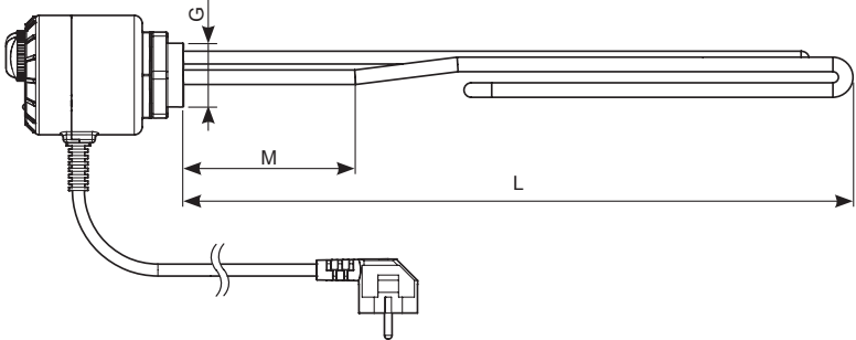
Рис. 9. Нагревательный модуль ME 1030.
