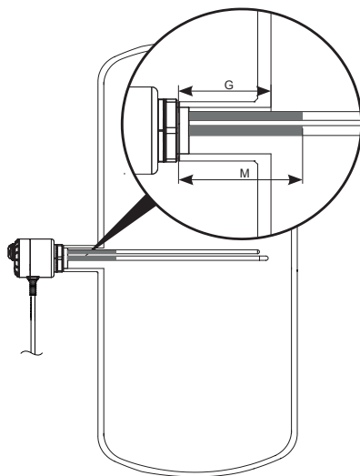
Рис. 3 Правильная глубина соединительного штуцера
