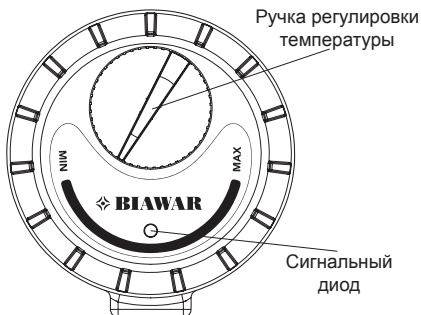
Рис. 7 Передняя часть корпуса нагревательного модуля ME 1030.
