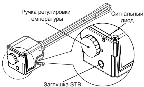
Рис. 8 Передняя часть корпуса нагревательных модулей ME 0040 / ME 1045 / ME 1060 / ME 1090 / ME 2090 / ME 2120 / ME 2180
