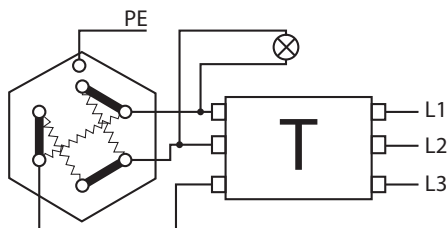
Ritning. 6 Elektriskt diagram ME 2120 - ME 2180.
