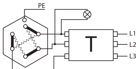
Rys. 6 Schemat elektryczny ME 2120 - ME 2180.
