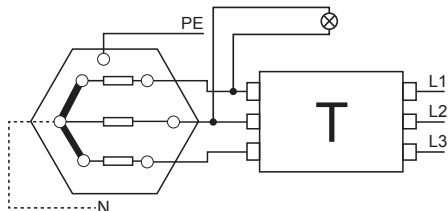
Ritning. 5 Elektriskt diagram ME 0040 - ME 2090.
