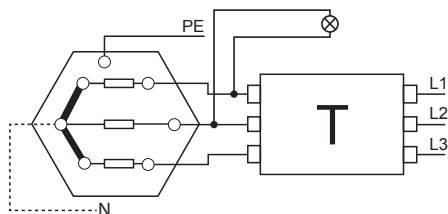
Рис. 5 Электрическая схема ME 0040 - ME 2090.
