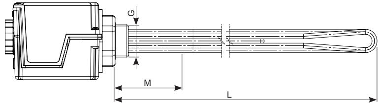
Fig. 10. ME 0040 / ME 1045 / ME 1060 / ME 1090 / ME 2090 / ME 2120 / ME 2180 heating module.
