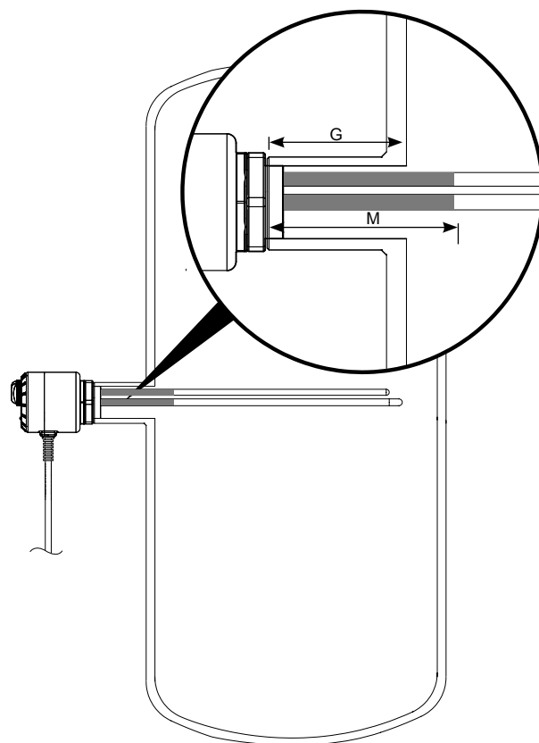
Рис. 3 Правильная глубина соединительного штуцера.
