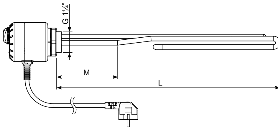
Rys. 8. Wymiary modułu grzejnego ME 0020 oraz ME 0030.
