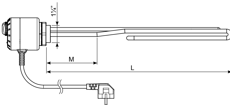
Рис. 8. Размеры нагревательного модуля ME 0020 и ME 0030.
