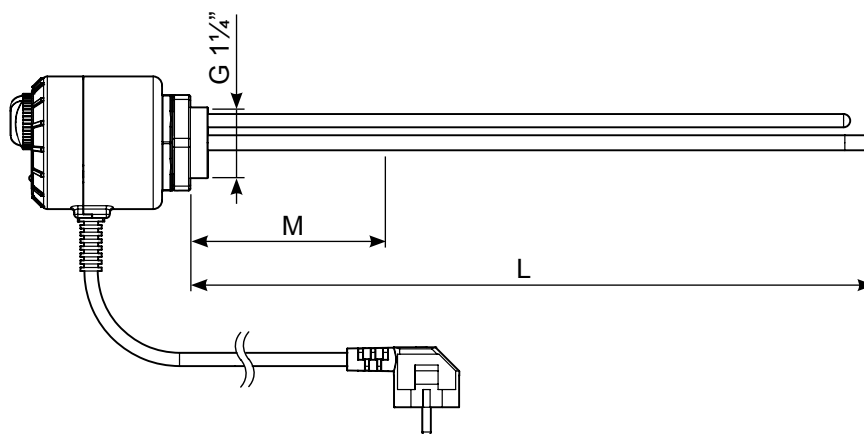
Rys. 7. Wymiary modułu grzejnego ME 0015.
