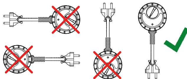
Rys. 4 Poprawny montaż modułu grzejnego.
