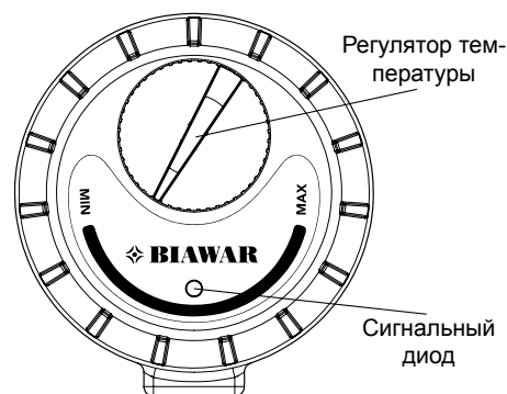
Рис. 5 передние корпуса нагревательного модуля.
