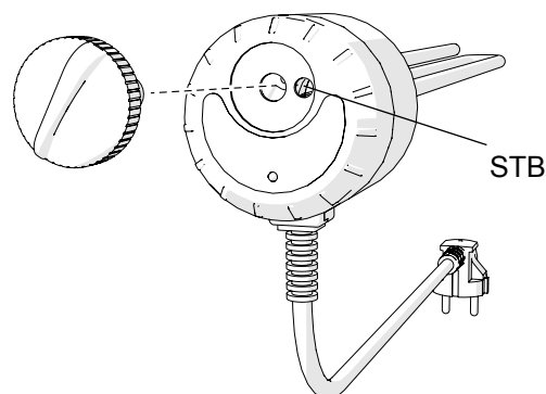
Rys. 6 Ogranicznik STB.
