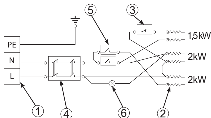
Rys. 8 Schemat elektryczny
