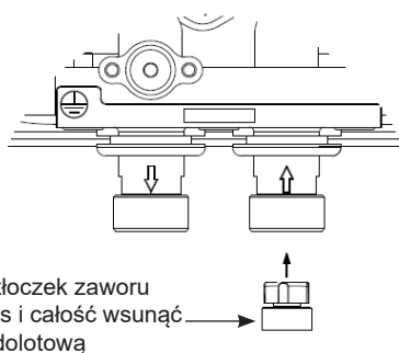
Rys. 10 Montaż zaworu zwrotnego
