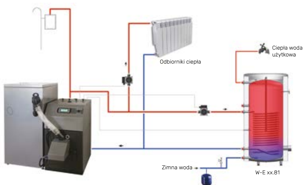
Przykładowy schemat instalacyjny z zasobnikiem W-E xx.81
