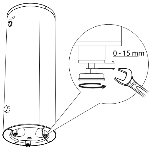
Rys. 4 Poziomowanie urządzenia.
