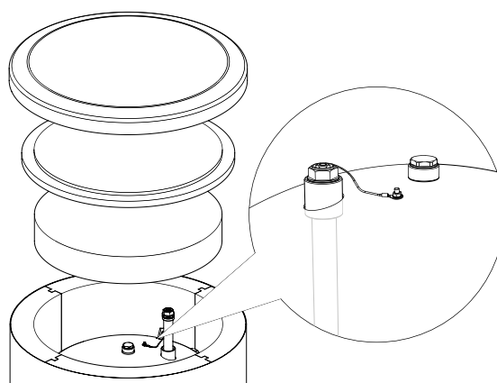
Rys. 10 Odizolowana ochronna anoda magnezowa.
