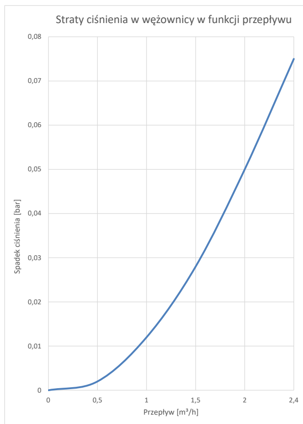
Rys. 20 Straty ciśnienia w węźnicy górnej W-E 500.82N
