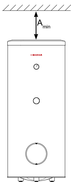
Rys. 6 Minimalna odległość do wymiany ochronnej anody magnezowej.
