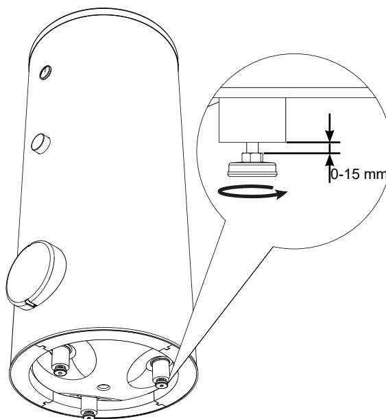
Rys. 7 Poziomowanie urządzenia.
