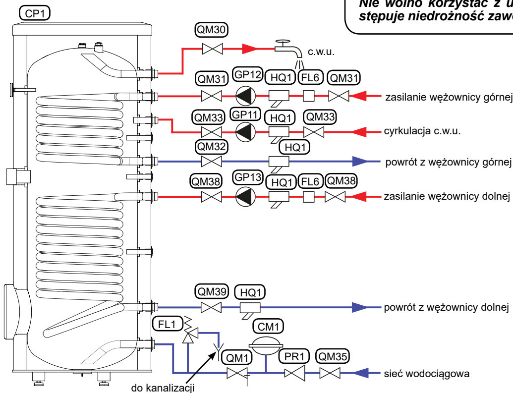
Rys. 9 Schemat instalacyjny zasobnika z dwoma węzownikami MEGA SOLAR.
