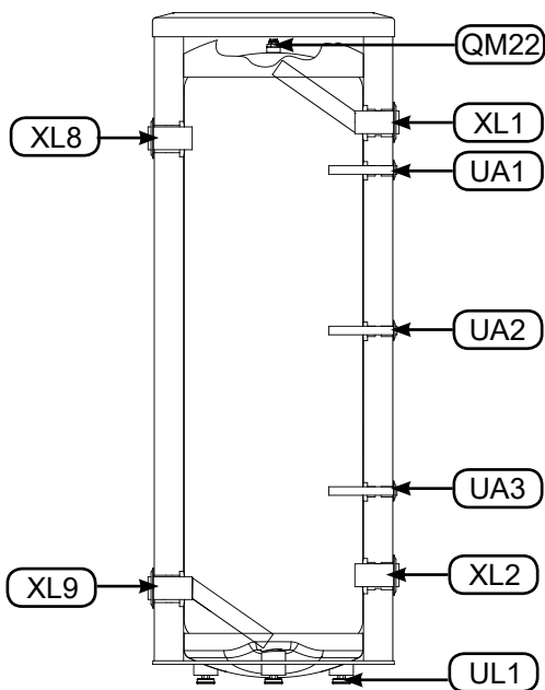
Rys. 4 Przekrój zbiornika BU-220.8 N.
