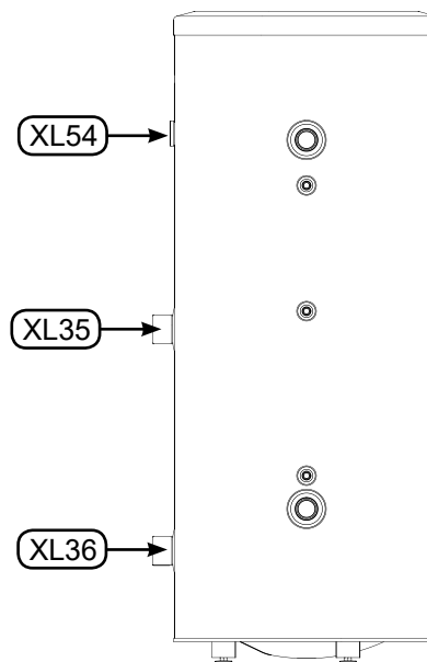
Rys. 7 Widok z boku zbiornika BU-300.8 N oraz BU-500.82 N.
