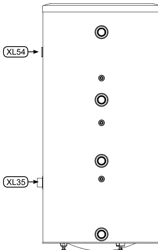
Rys. 9 Widok z boku zbiornika BU-750-1000.8 N.
