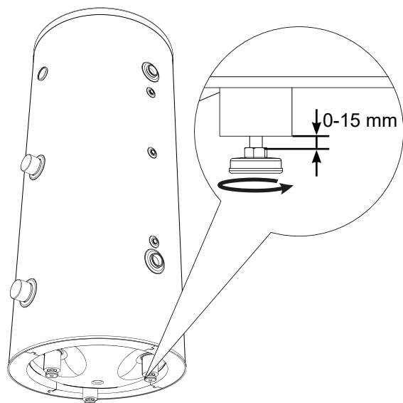
Rys. 10 Poziomowanie urządzenia.
