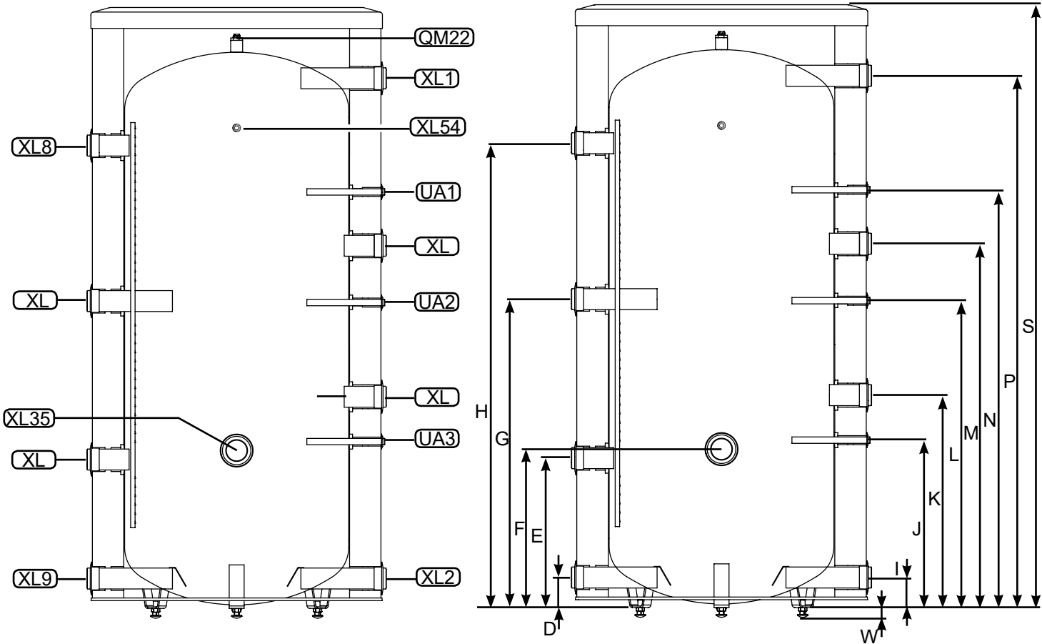
Rys. 17 Wymiary zbiorników buforowych BU-750 - 1000.8
