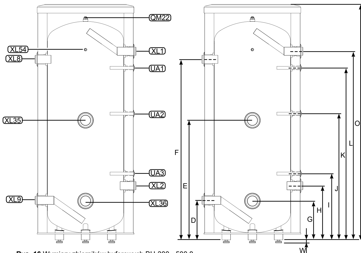
Rys. 16 Wymiary zbiorników buforowych BU-300 - 500.8
