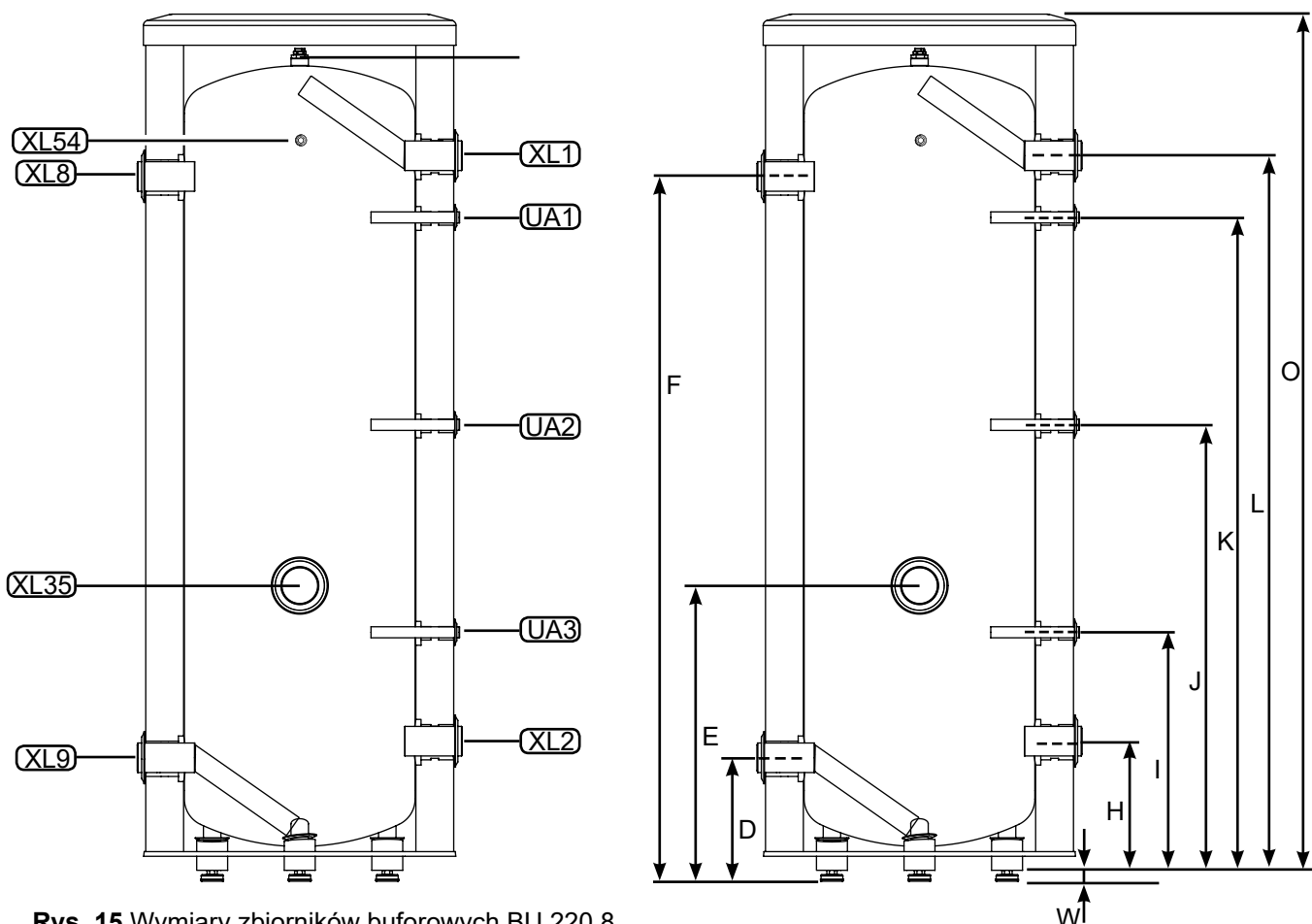
Rys. 15 Wymiary zbiorników buforowych BU 220.8
