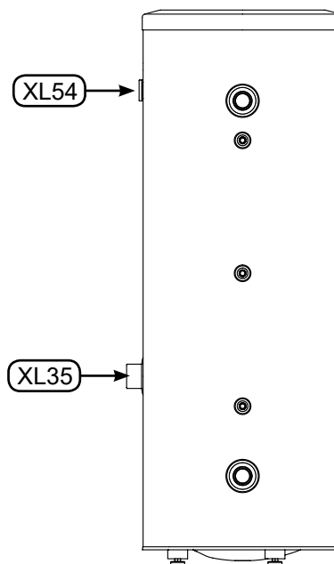
Rys. 5 Widok z boku zbiornika BU-220.8 N.
