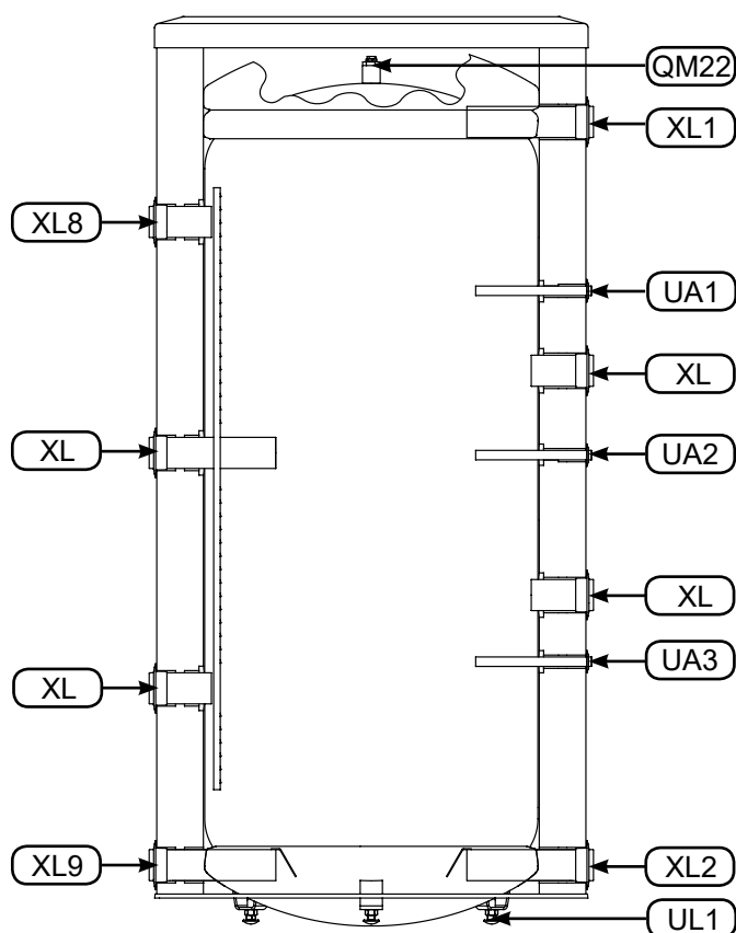
Rys. 8 Przekrój zbiornika BU-750-1000.8 N.
