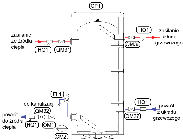
Rys. 13 Schemat instalacyjny zbiornika buforowego w instalacji zamkniętej.
