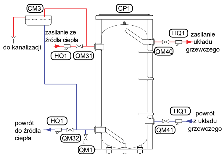
Rys. 12 Schemat instalacyjny zbiornika buforowego w instalacji otwartej.
