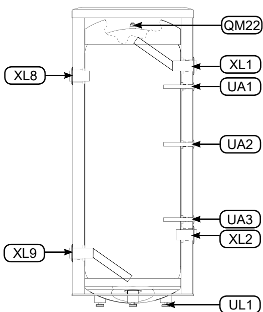
Rys. 6 Przekrój zbiornika BU-300.8 N oraz BU-500.8 N.
