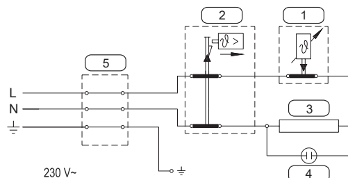
Rys. 10 Schemat instalacji elektrycznej podgrzewacza GT 5/10/15 U, GT 5/10/15 O.
