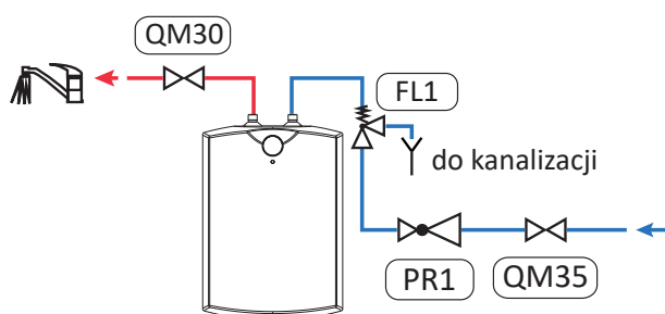
Rys. 8 Schemat instalacyjny podgrzewaczy podumywalkowych GT 5/10/15 U.
