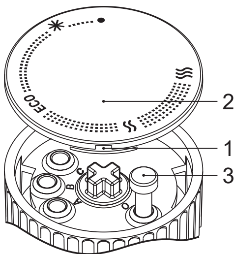
Rys. 11 Ograniczenie nastawy maksymalnej temperatury wody w ogrzewaczu.
