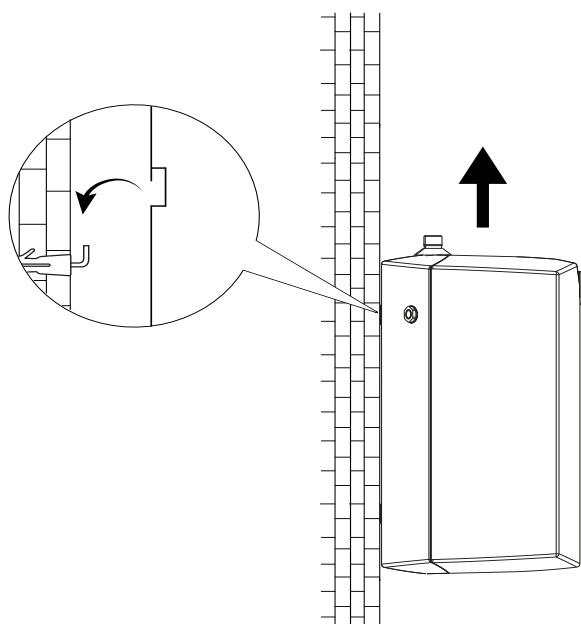
Rys. 5 Montaż podgrzewaczy podumywalkowych (GT 5/10/15 U).
