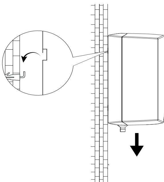
Rys. 6 Montaż podgrzewaczy nadumywalkowych (GT 5/10/15 O).
