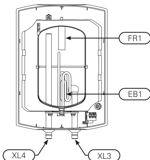
Rys. 4 Przekrój podgrzewacza GT 5/10/15 O nadumywalkowego
