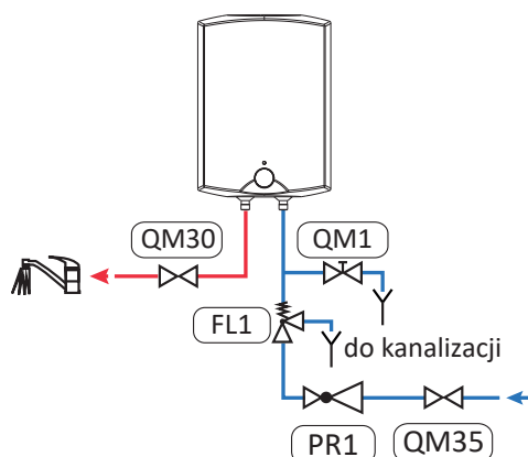
Rys. 8 Schemat instalacyjny podgrzewaczy podumywalkowych GT 5/10/15 U.
