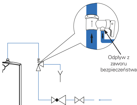
Rys. 7 Zalecana pozycja zaworu bezpieczeństwa na przykładzie podgrzewacza podumywalkowego.
