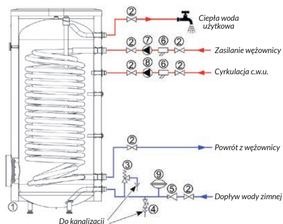
Rys. 1. Schemat instalacyjny zasobnika W-E 300/400/500.81 PC N.
