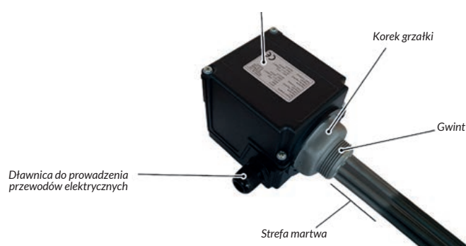
Tabliczka znamionowa
