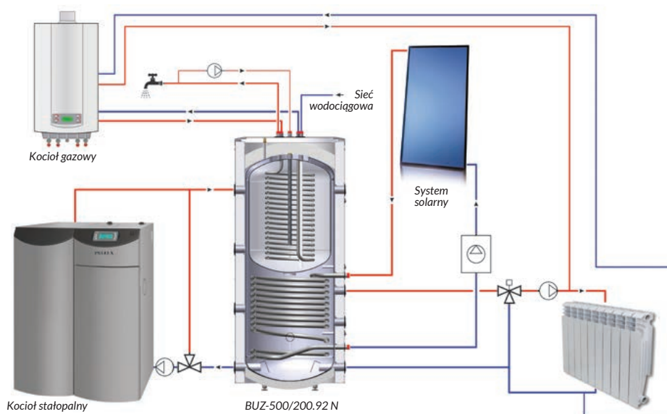
Rys. 1. Przykładowy schemat instalacyjny ze zbiornikiem multiwalentnym BUZ-500/200.92 N
