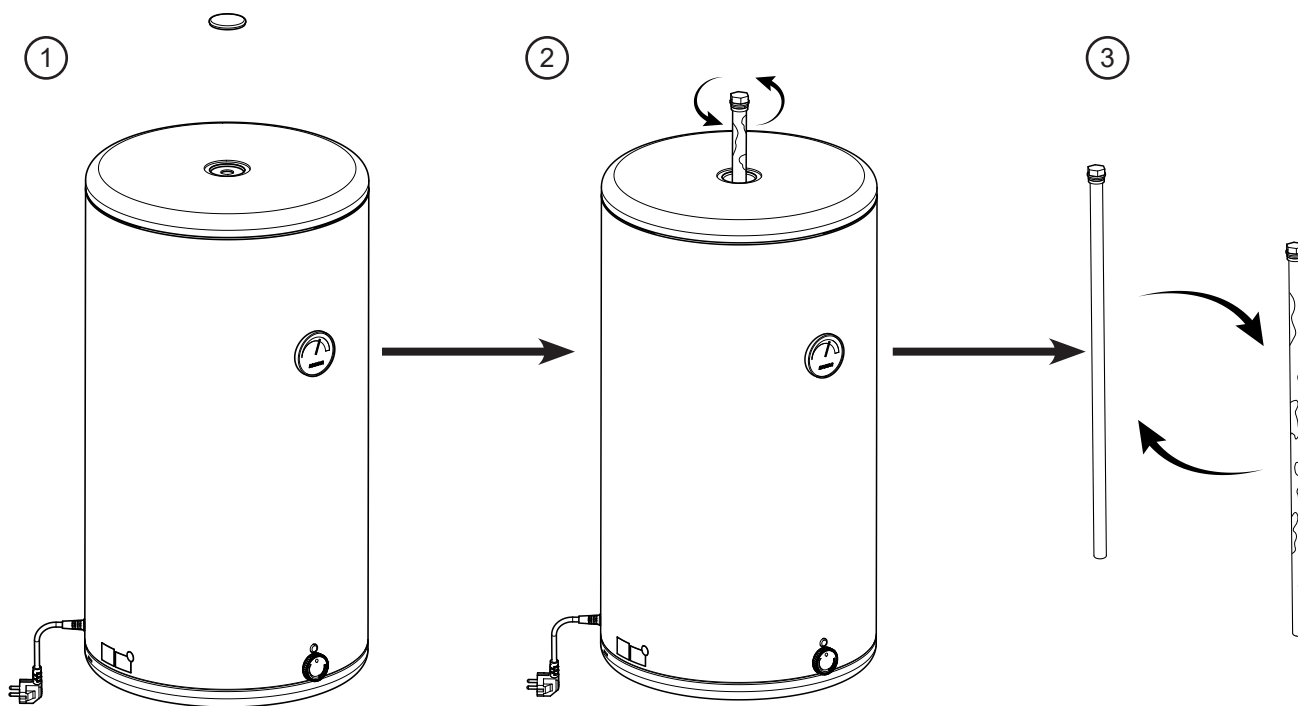
Rys. 12 Wymiana ochronnej anody magnezowej
