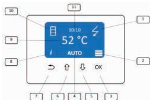
Rys. 17 – Wyświetlacz (sterownik)
