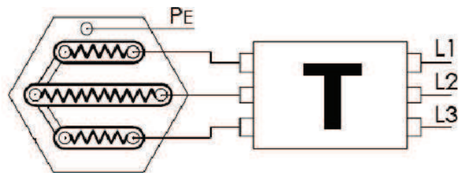
Schemat podłączenia
