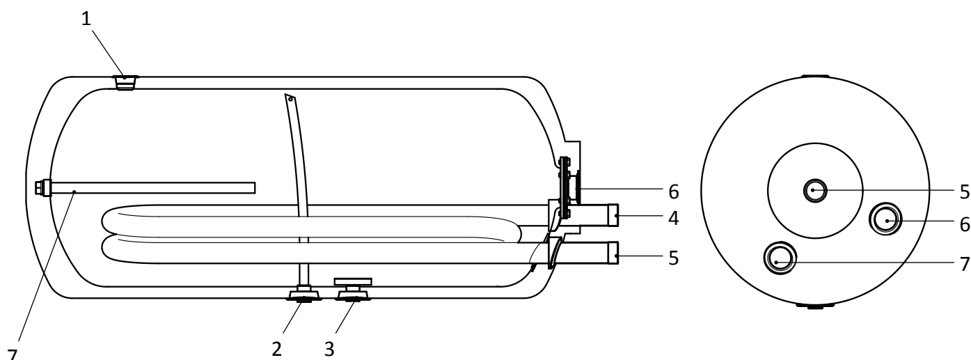
Rys. 2 Przekrój zasobnika W-E 120-140.25 Plus.
