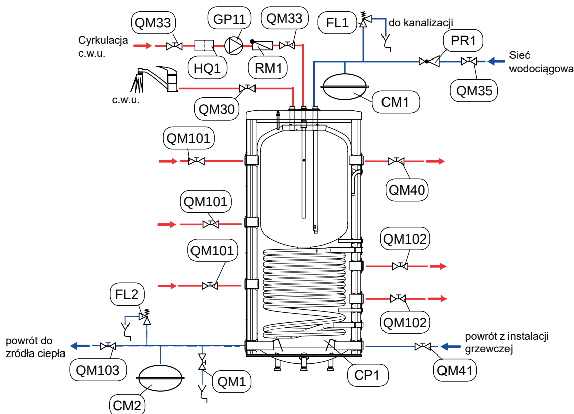
Rys. 10 Schemat instalacyjny (układ zamknięty).
