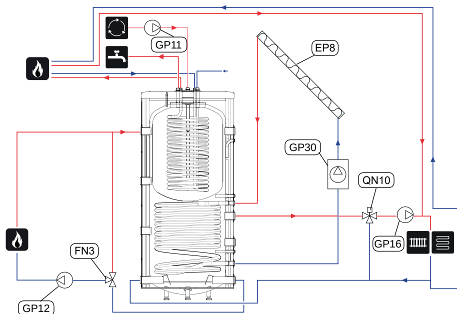
Rys. 12 Schemat instalacyjny zbiornika BUZ- 400/15-.92 N BUZ- 500/200.92 N.
