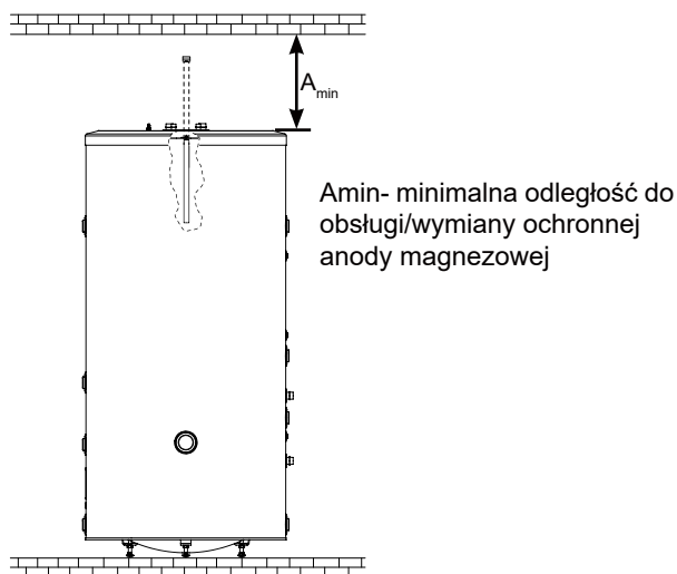
Rys. 5 Minimalna odległość do obsługi / wymiany odizolowanej magnezowej anody ochronnej
