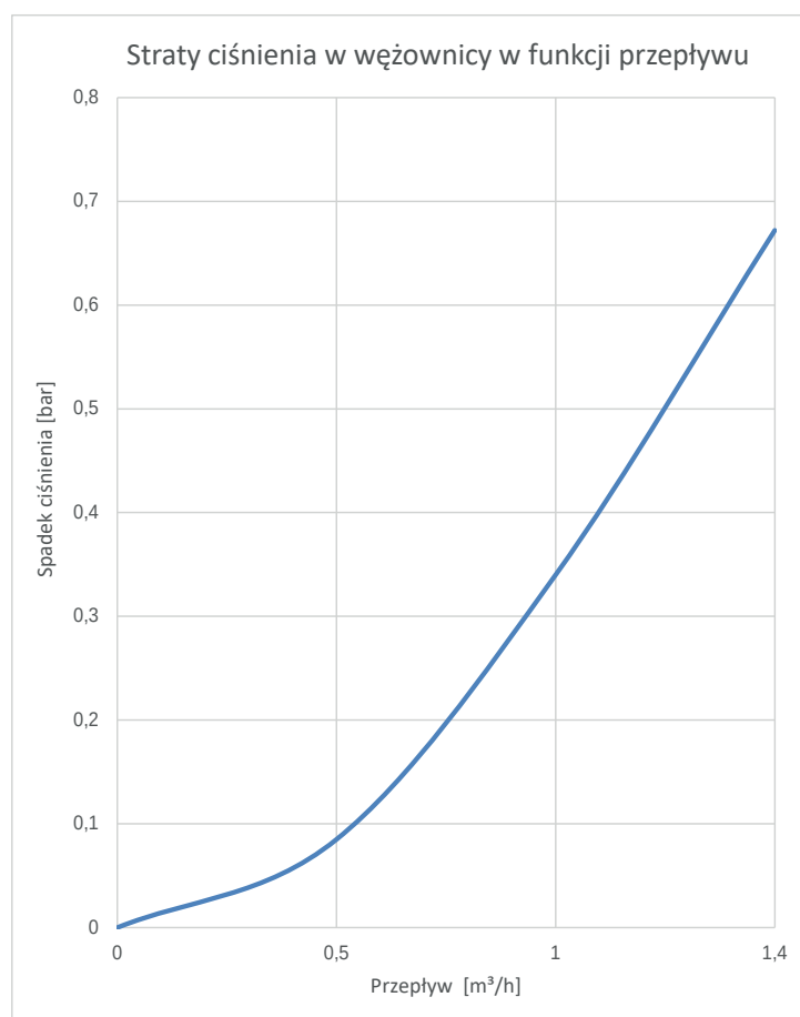
Rys. 20 Staty ciśnienia w wewnętrznej węzownicy w zbiorniku BUZ 500/200.92 N
