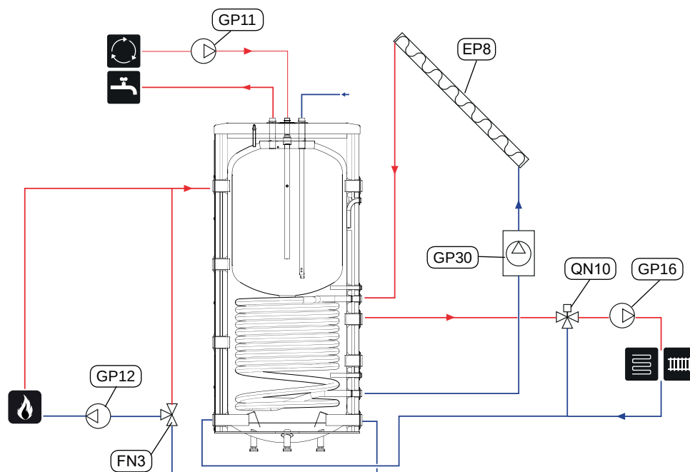
Rys. 11 Schemat instalacyjny zbiornika BUZ- 400/15-.91 N BUZ- 500/200.91 N.
