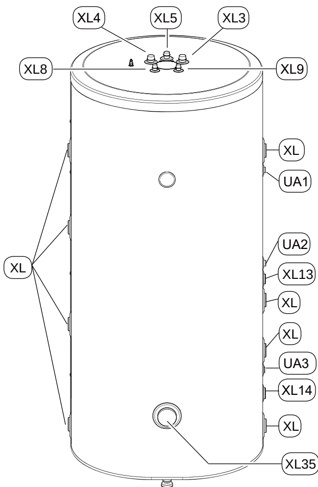
Rys. 4 BUZ - 500/200.92N
