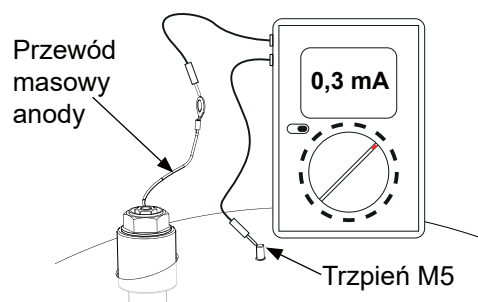
Rys. 15 Pomiar natężenia stałego prądu ochronnego
