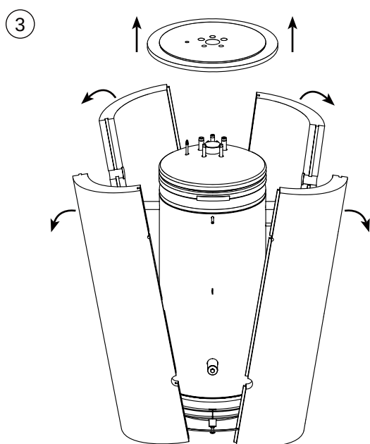
Rys. 7 Demontaż obudowy
