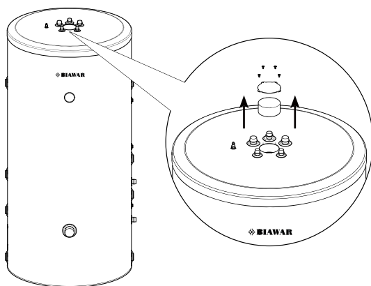
Rys. 14 Demontaż zaślepki pokrywę górnej.
