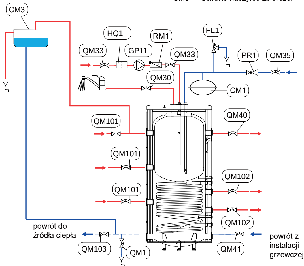
Rys. 9 Schemat instalacyjny (układ otwarty).
