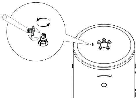
Rys. 13 Odpowietrzanie zbiornika zewnętrznego.
