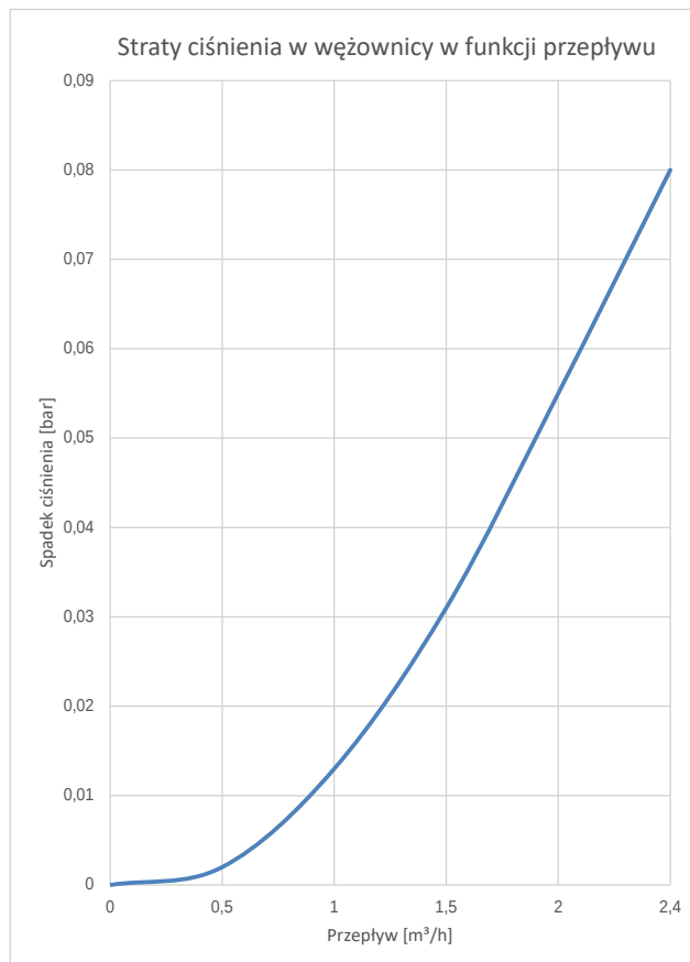
Rys. 17 Staty ciśnienia w węźownicy w zbiorniku BUZ 400/150.91 N oraz węźownicy dolnej w BUZ 400/150.92 N.
