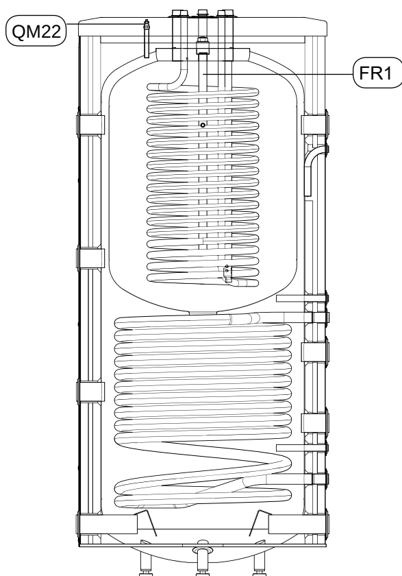
Rys. 2 Budowa BUZ-400/150.92N; BUZ -500/200.92N
