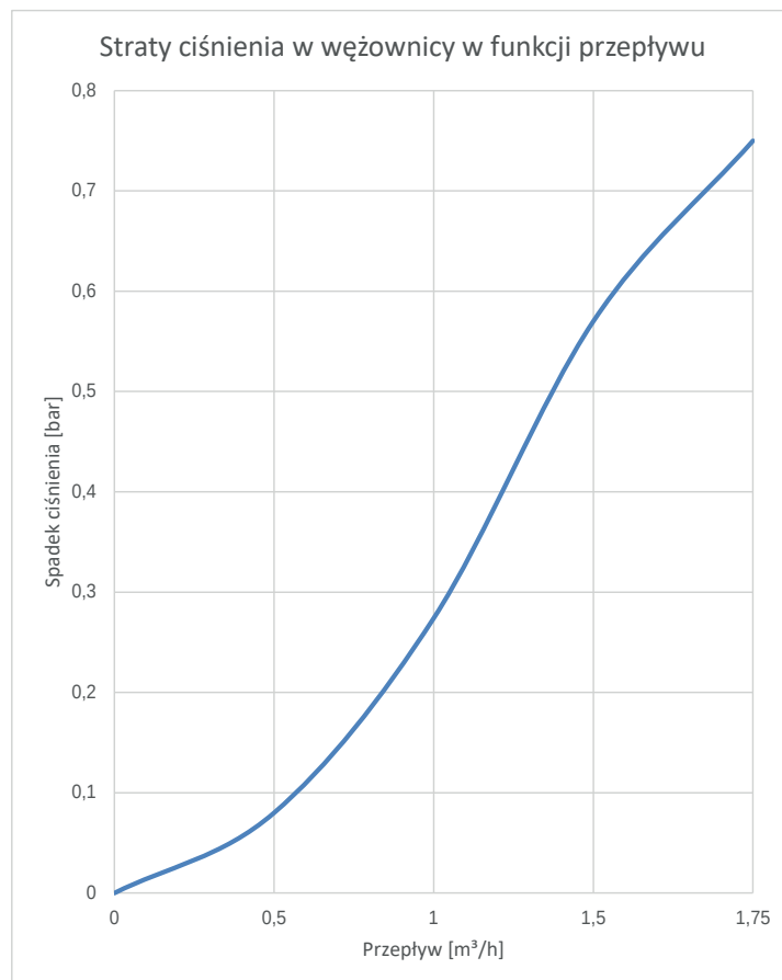
Rys. 19 Staty ciśnienia w wewnętrznej węzownicy w zbiorniku BUZ 400/150.92 N
