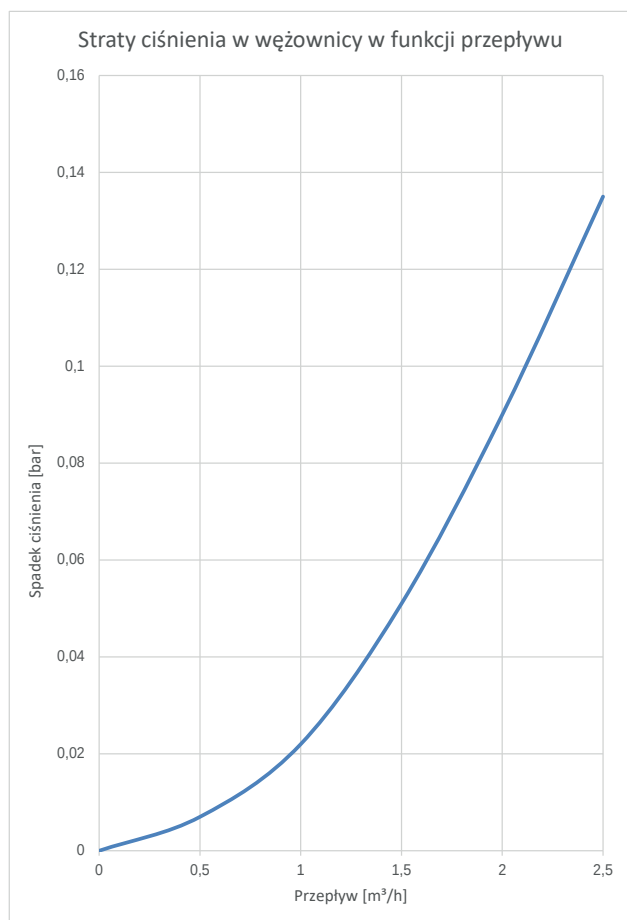
Rys. 18 Staty ciśnienia w węźownicy w zbiorniku BUZ 500/200.91 N oraz węźownicy dolnej w BUZ 500/200.92 N.
