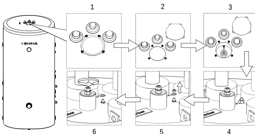
Rys. 16 Wymiana ochronnej anody magnezowej.
