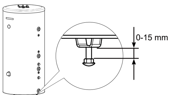
Rys. 6 Poziomowanie urządzenia.
