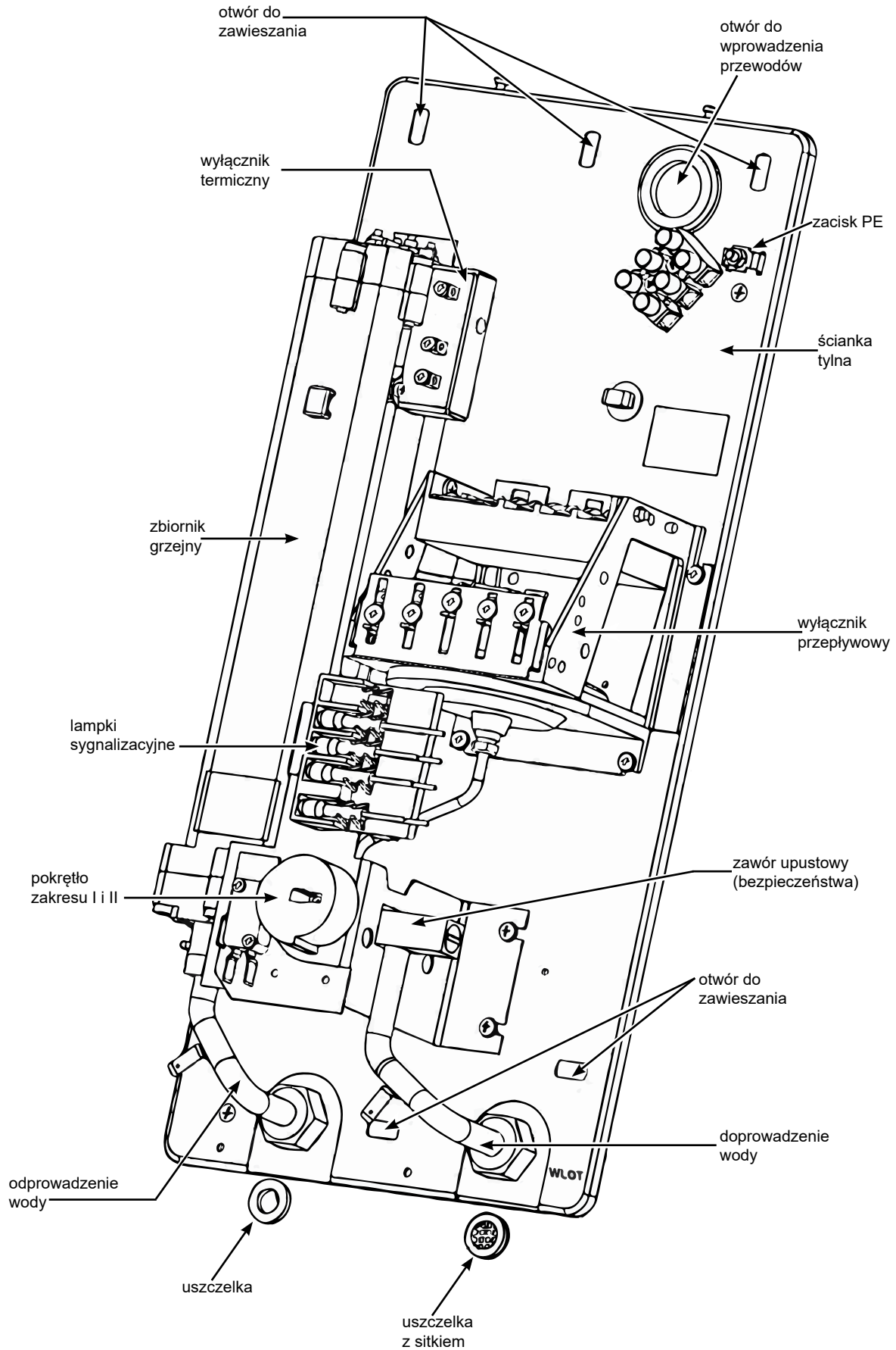
Rys.5 Budowa podgrzewacza
