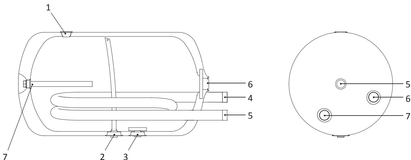
Rys. 2 Przekrój zasobnika W-E 80-140.25 Plus.
