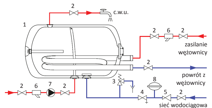
Rys. 5 Schemat podłączenia z cyrkulacją.
