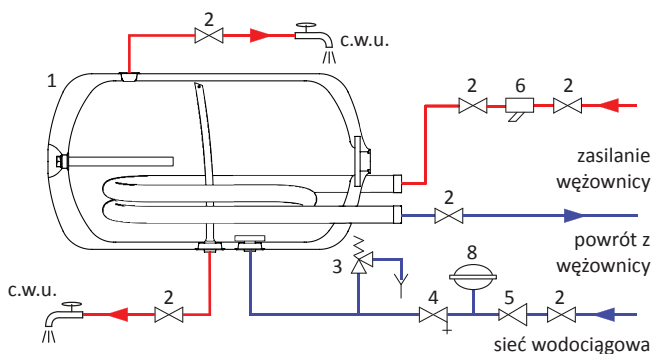
Rys. 4 Schemat podłączenia bez cyrkulacji.
