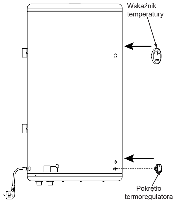
Rys. 9 Montaż pokrętła termoregulatora i wskaźnika temp.
