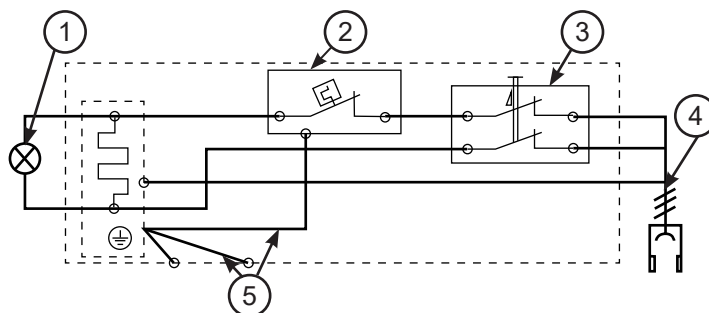
Rys. 8 Schemat instalacji elektrycznej podgrzewacza Classic
