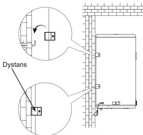
Rys. 5 Zawieszenie podgrzewacza.
