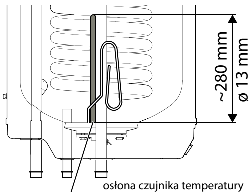
Rys. 8 Osłona czujnika temperatury VIKING PLUS E100, E150
