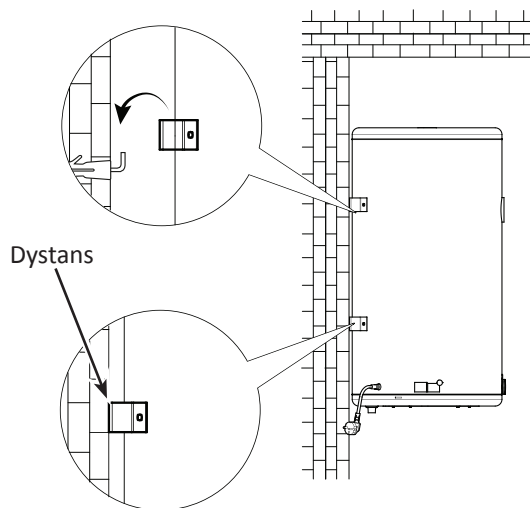
Rys. 4 Zawieszenie podgrzewacza.
