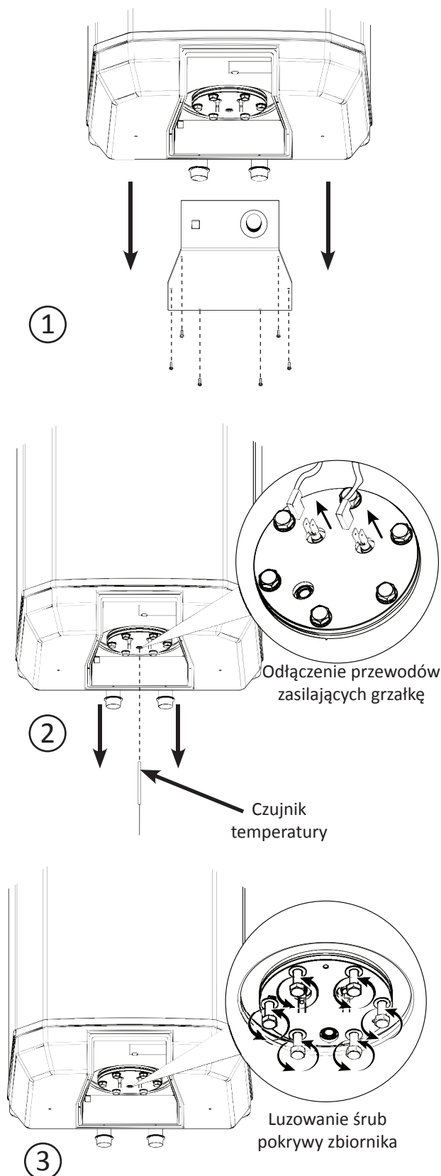
Rys. 9 Opróżnianie zbiornika podgrzewacza VIKING E
