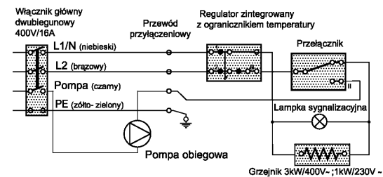
Rys.2. Schemat elektryczny rozmieszczenia automatyki
