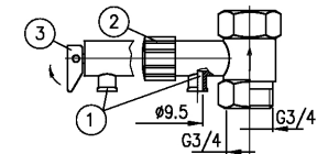
Rys.3. Zawór bezpieczeństwa (przykładowy)
