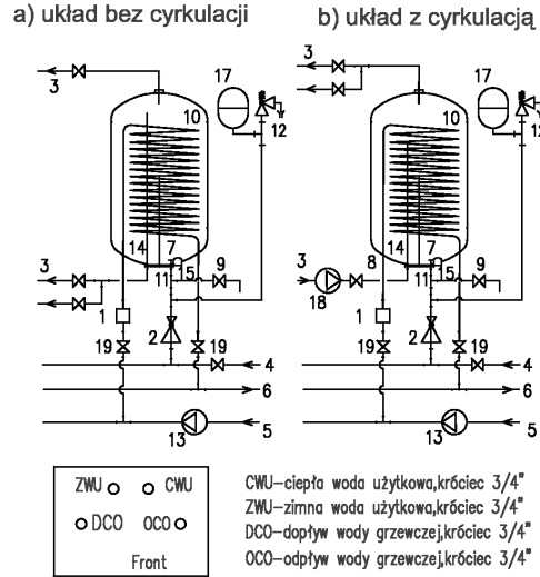
Rys.6 Schemat instalacyjny wymiennika W-E 60/200.7
